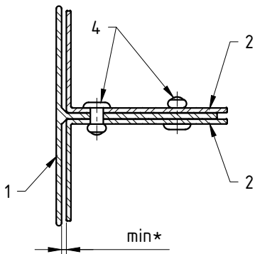
Метод удлинения (наращивания) профилей MFT-T и MFT-Ta
