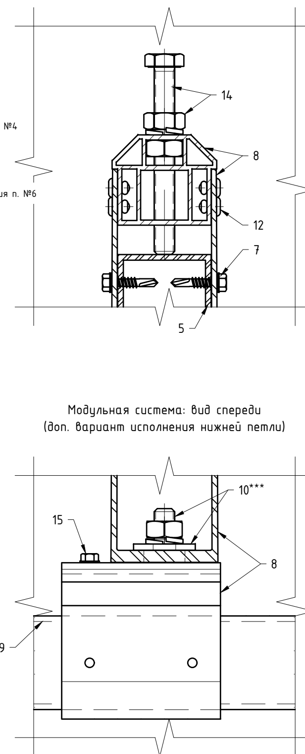
Модульная система: вид спереди (показано с регулировочным комплектом M12)
