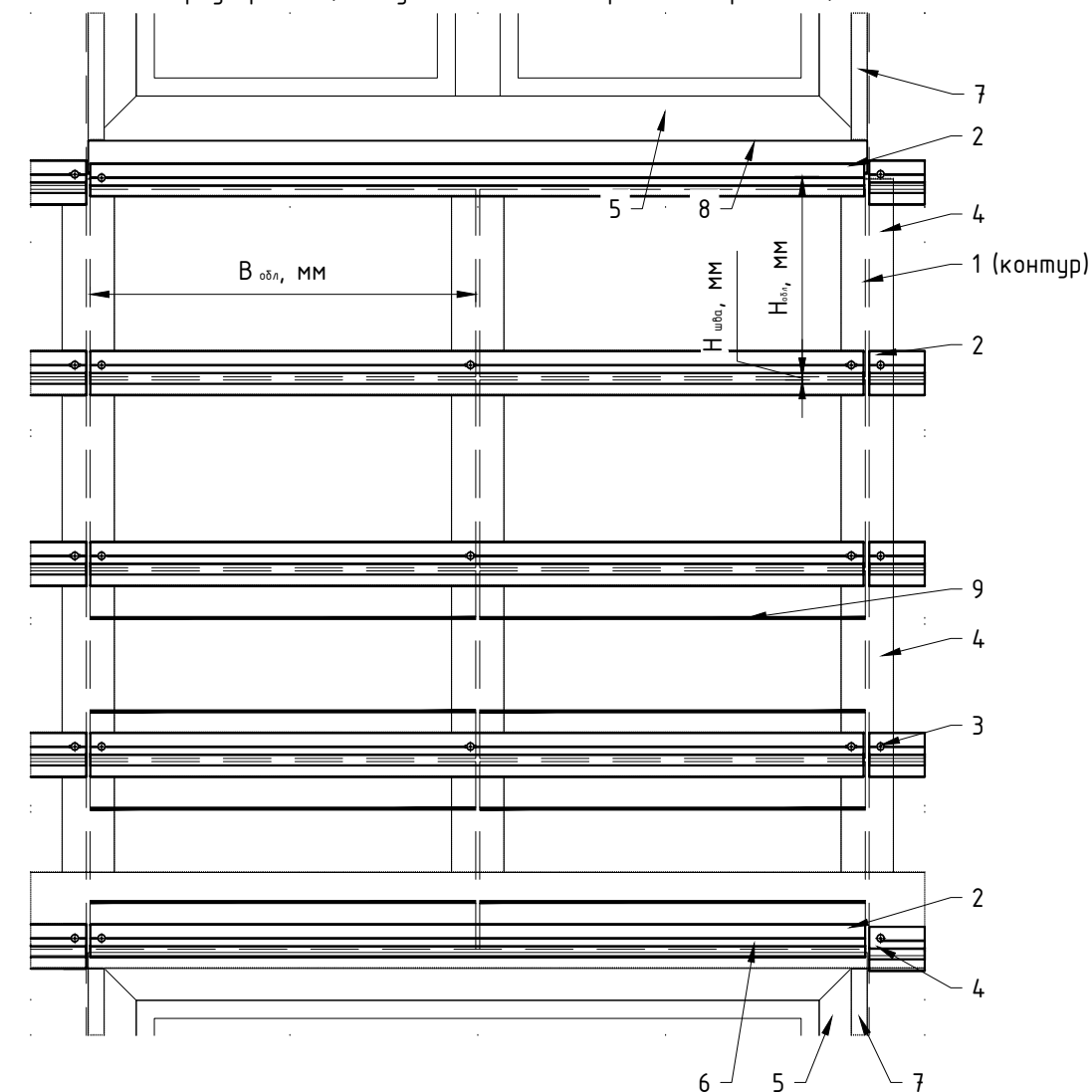
Для терракоты с креплением на алюминиевых клеммер-шинах NBK: в верху проема (между смежными по вертикали проемами)
