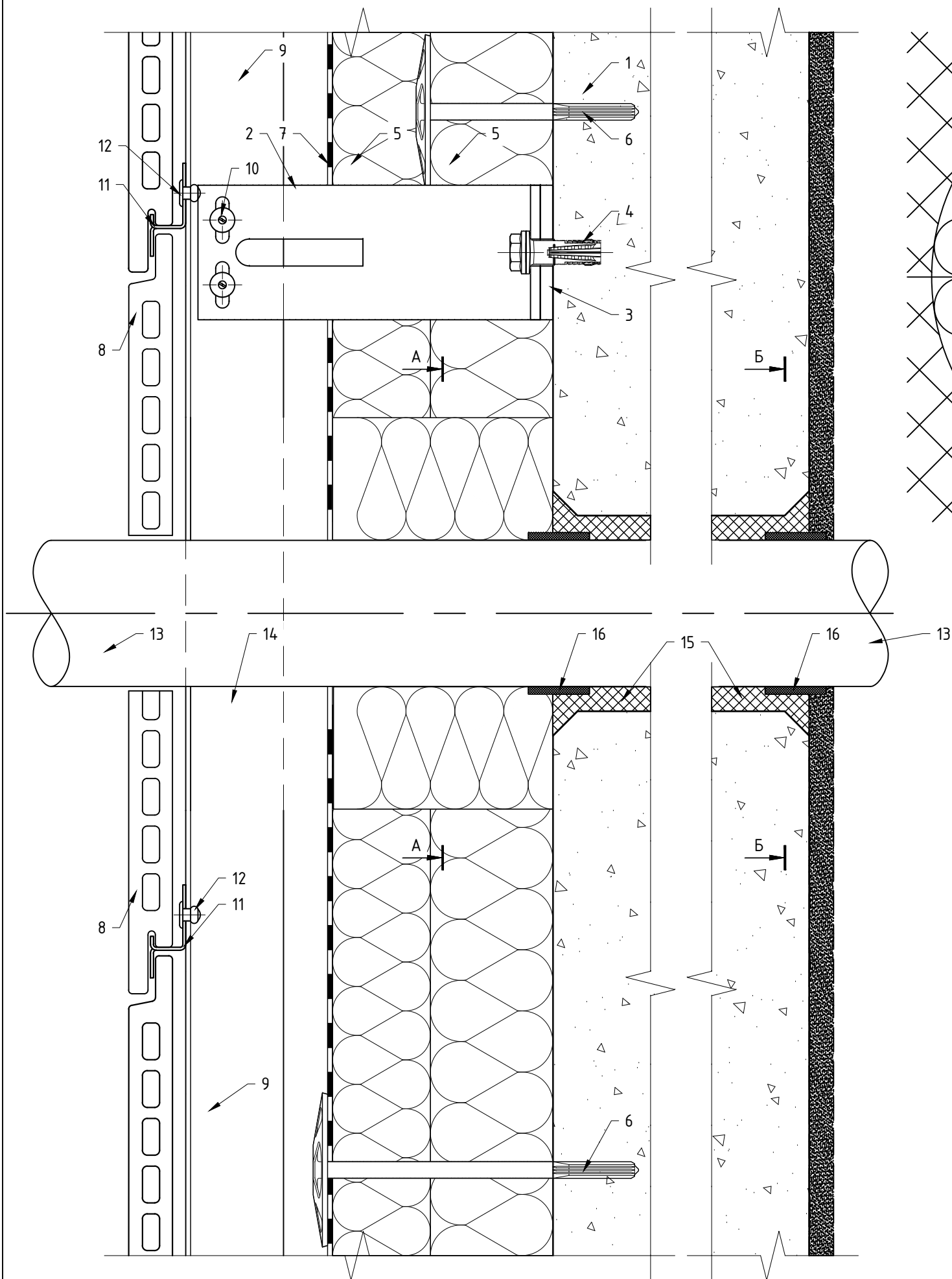
7.11. Ввод коммуникаций: элементы "Light", вертикальная схема расположения элементов системы, крепление с помощью кляммера MFT-CT StS.
