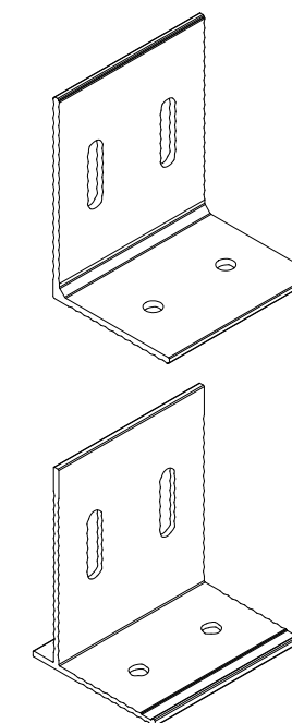
Пример детали обеспечения подвижного соединения
