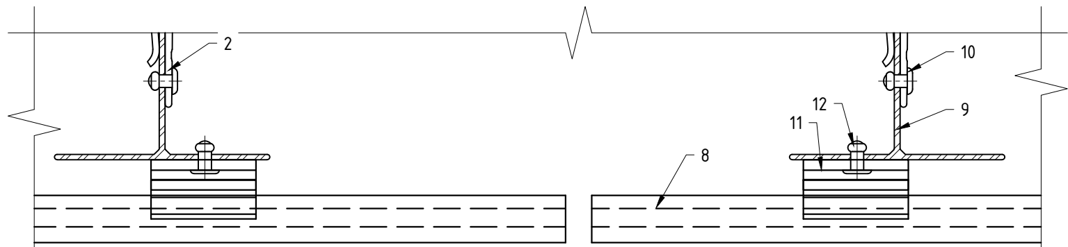
Вариант устройства деформационного шва с кляммерами MFT-NBK
