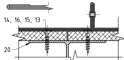
Сечение Б-Б
