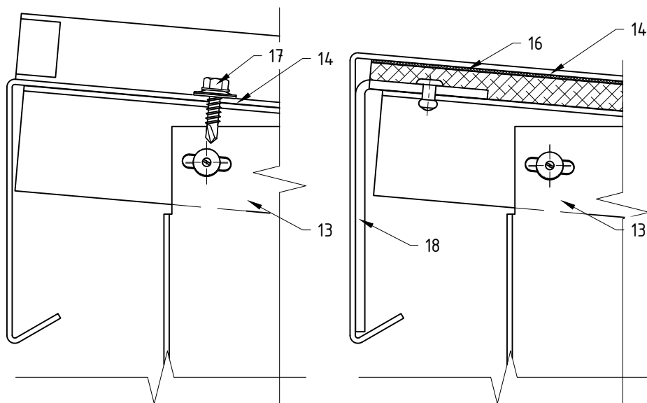
Вариант крепления парапетной крышки №2, №3.
