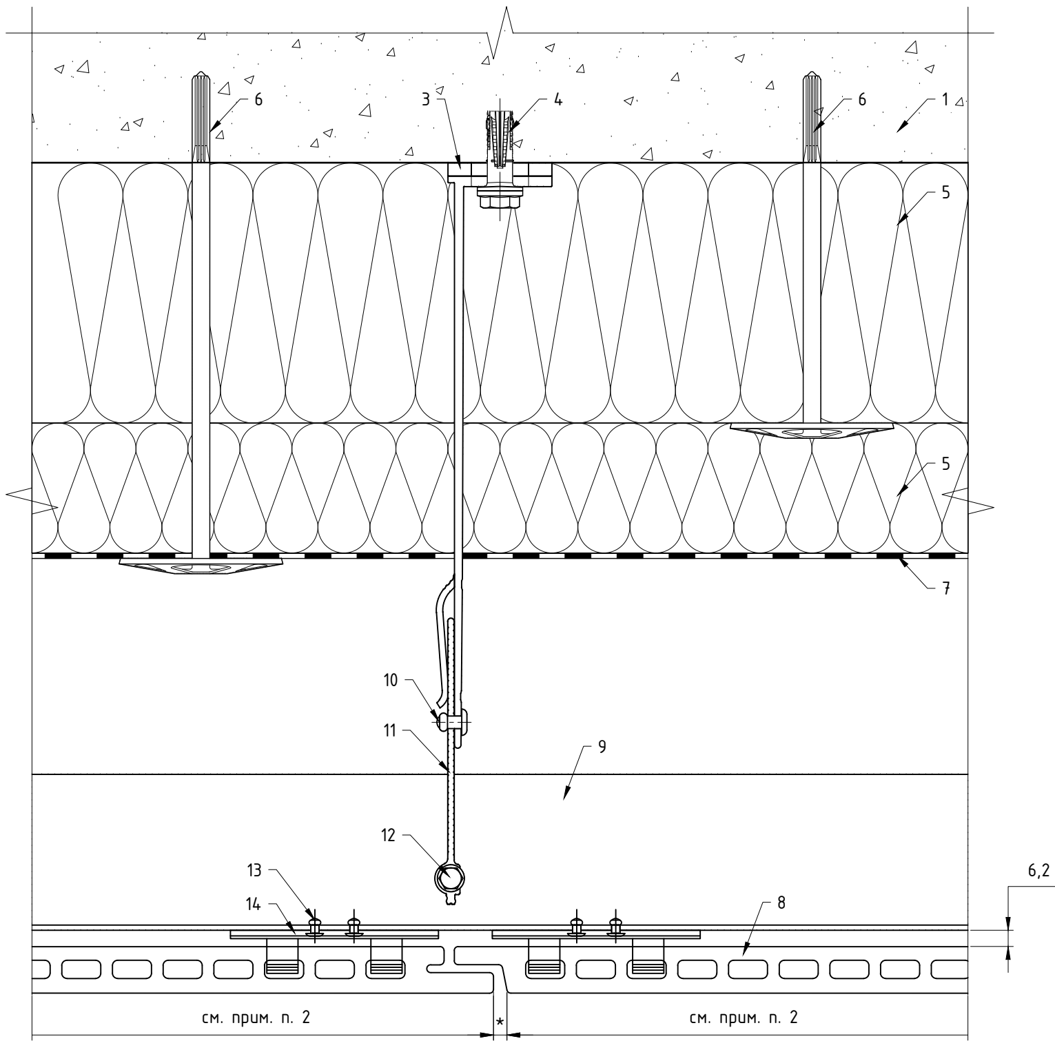
Горизонтальный разрез: элементы "Light", горизонтальная схема расположения элементов системы, крепление с помощью кляммера MFT-CT StS
