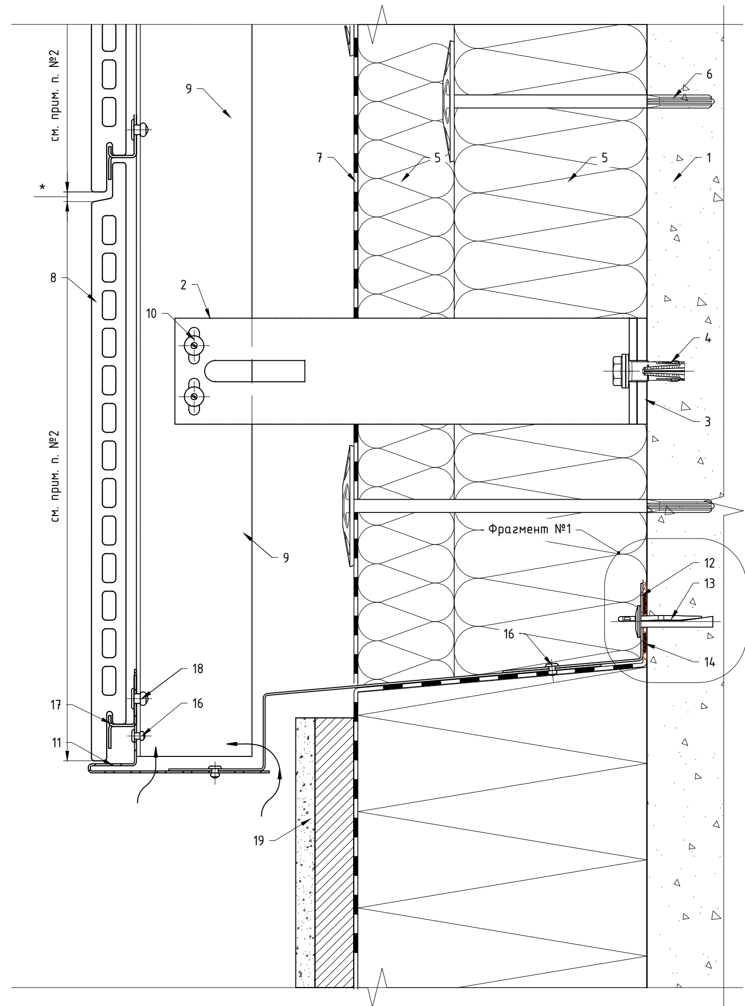
Примыкание к цоколю: вариант №3, вертикальная схема расположения элементов системы.
