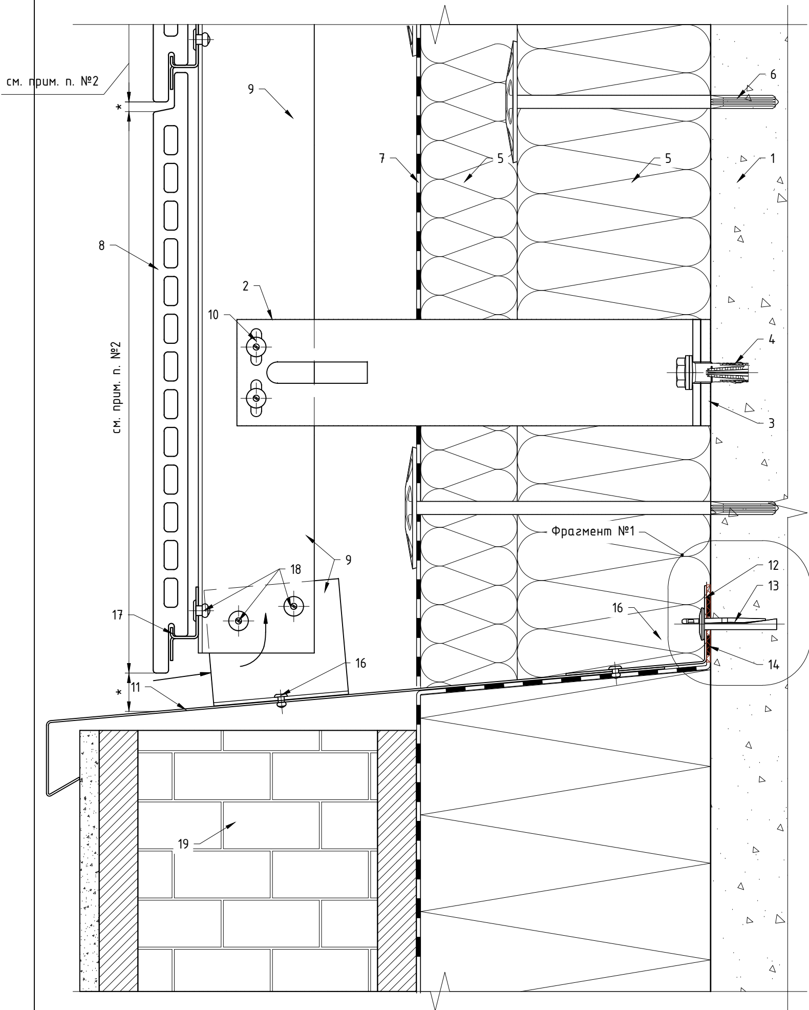
Примыкание к цоколю: вариант №2, вертикальная схема расположения элементов системы.
