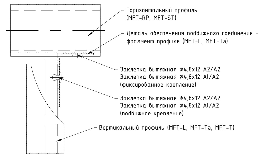
Узел №2 (увеличено)
