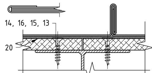
Сечение А-А (вар. 1, вар.2)
