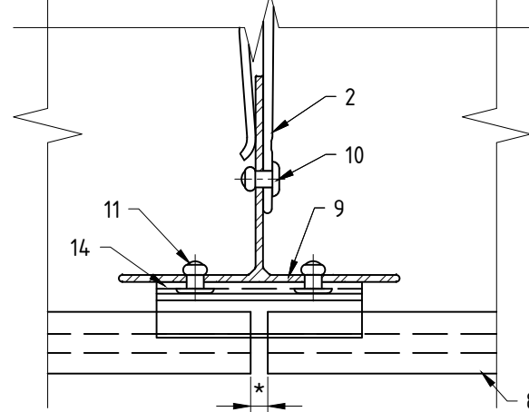
Фрагмент №1 (вариант применения кляммеров MFT-CTM 16,3 SPR)
