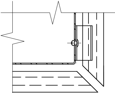
Фрагмент 1 (вариант запила терракоты)
