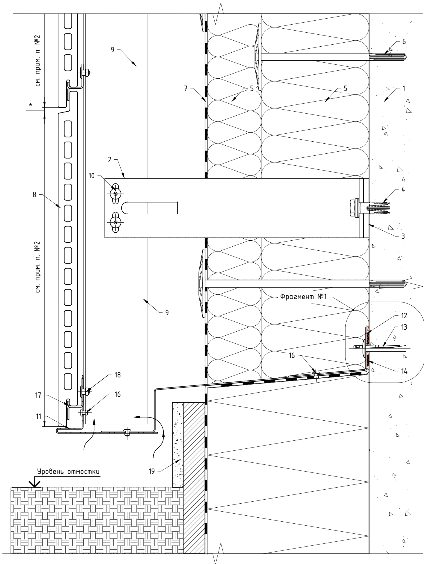
Примыкание к цоколю: вариант №4, вертикальная схема расположения элементов системы.
