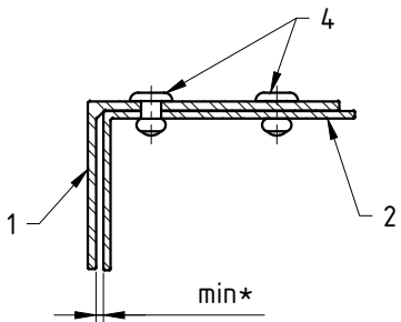
Метод удлинения (наращивания) профиля MFT-L
