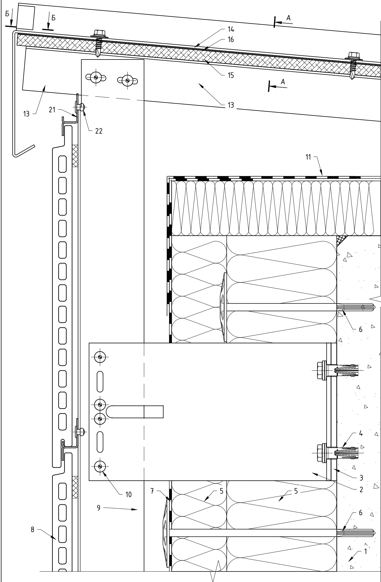
Сечение Б-Б
