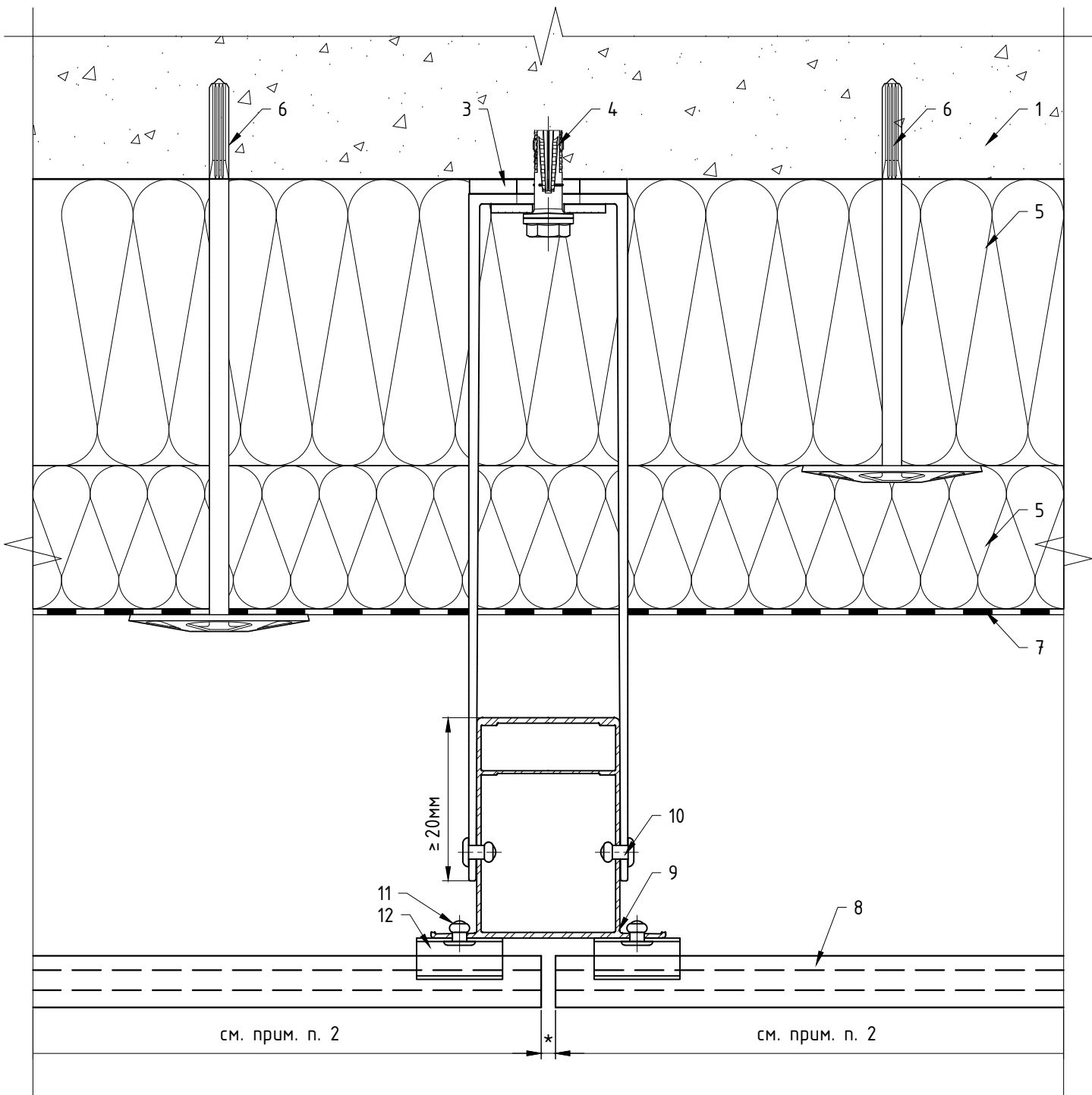
Горизонтальный разрез: элементы "Неву", крепление с помощью кляммера MFT-CT StS
