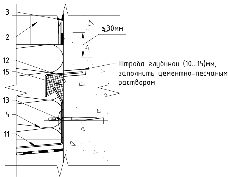
Крепление отлива к строительному основанию: вариант №2
