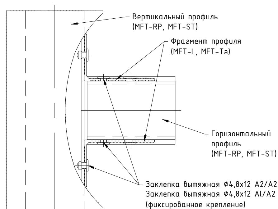
Узел №1 (увеличено)
