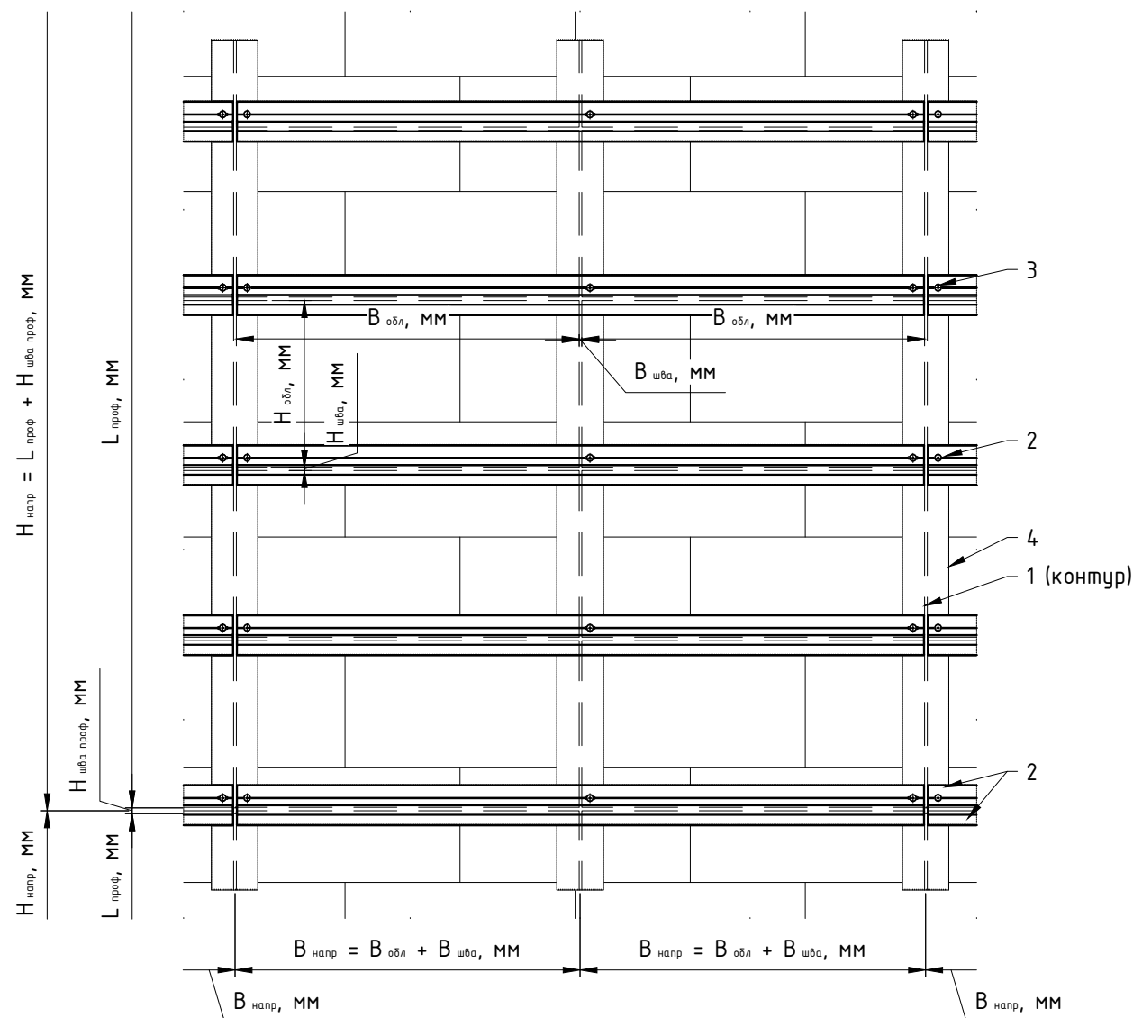
Для терракоты с креплением на алюминиевых клеммер-шинах NBK: рядовая зона (вне пожароопасных зон)
