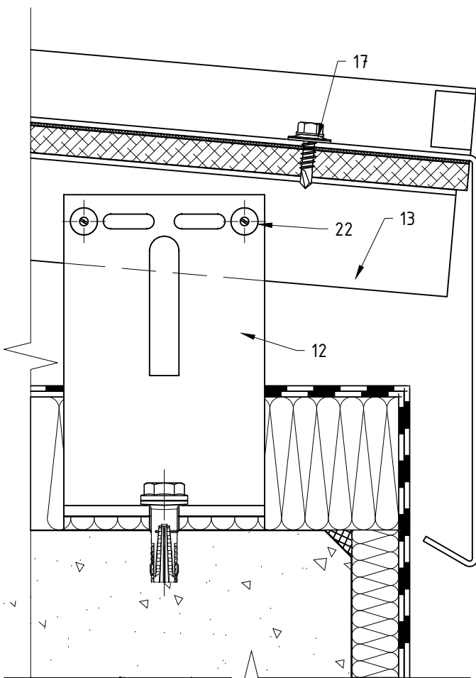
Сечение А-А (вар. 1, вар.2)
