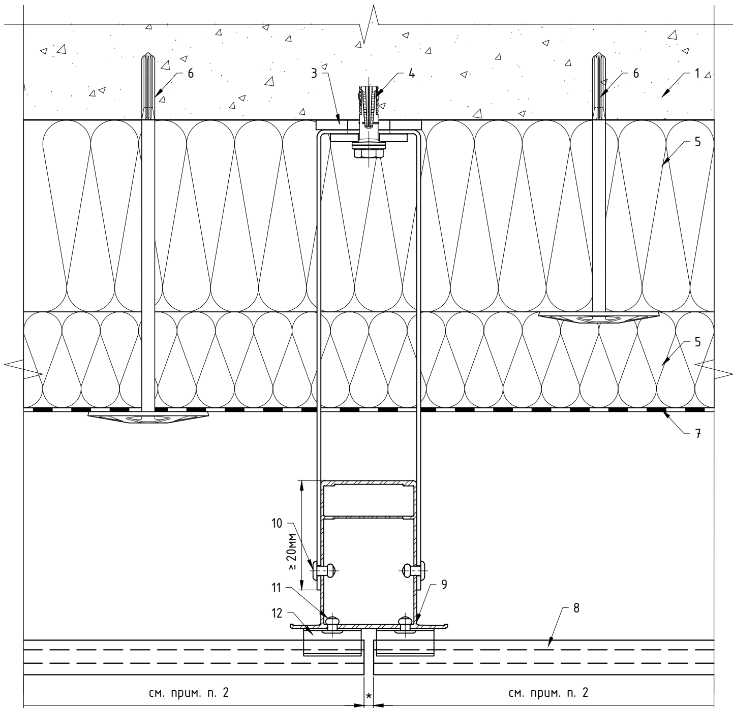
Горизонтальный разрез: элементы "Heavy", крепление с помощью кляммера MFT-CT StS
