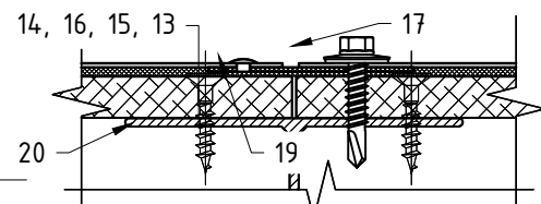
Сечение А-А (вар. 3)
